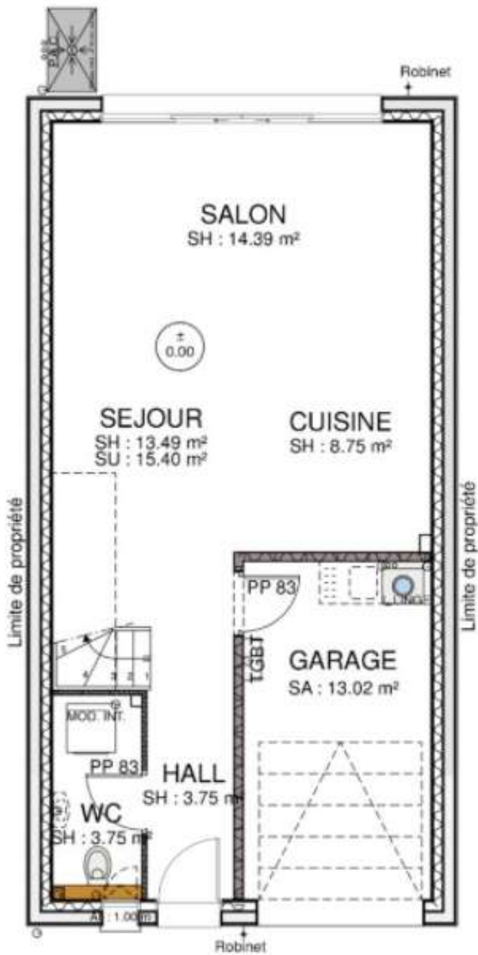
Plan RDC
